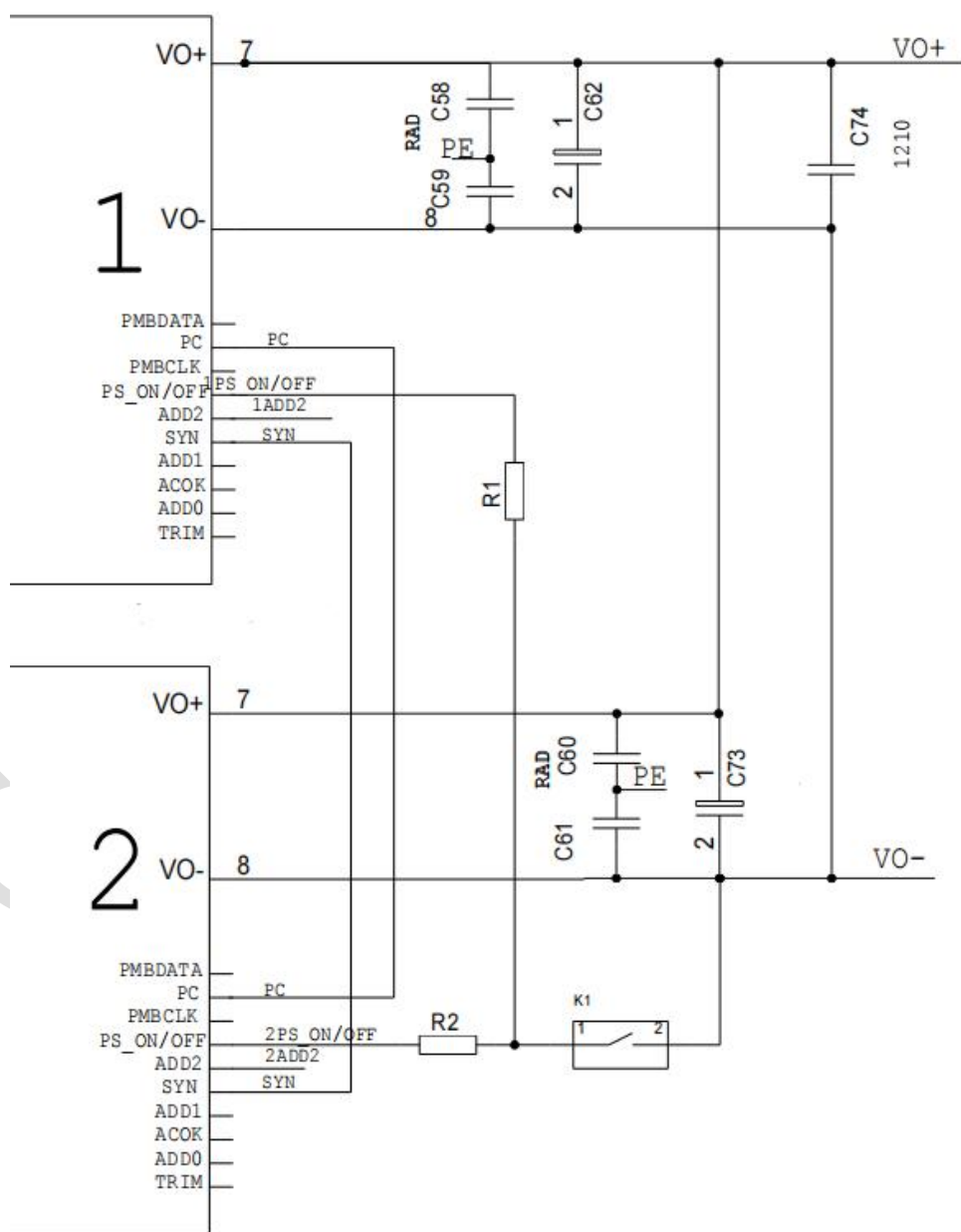
图 12 模块并联使用连接
